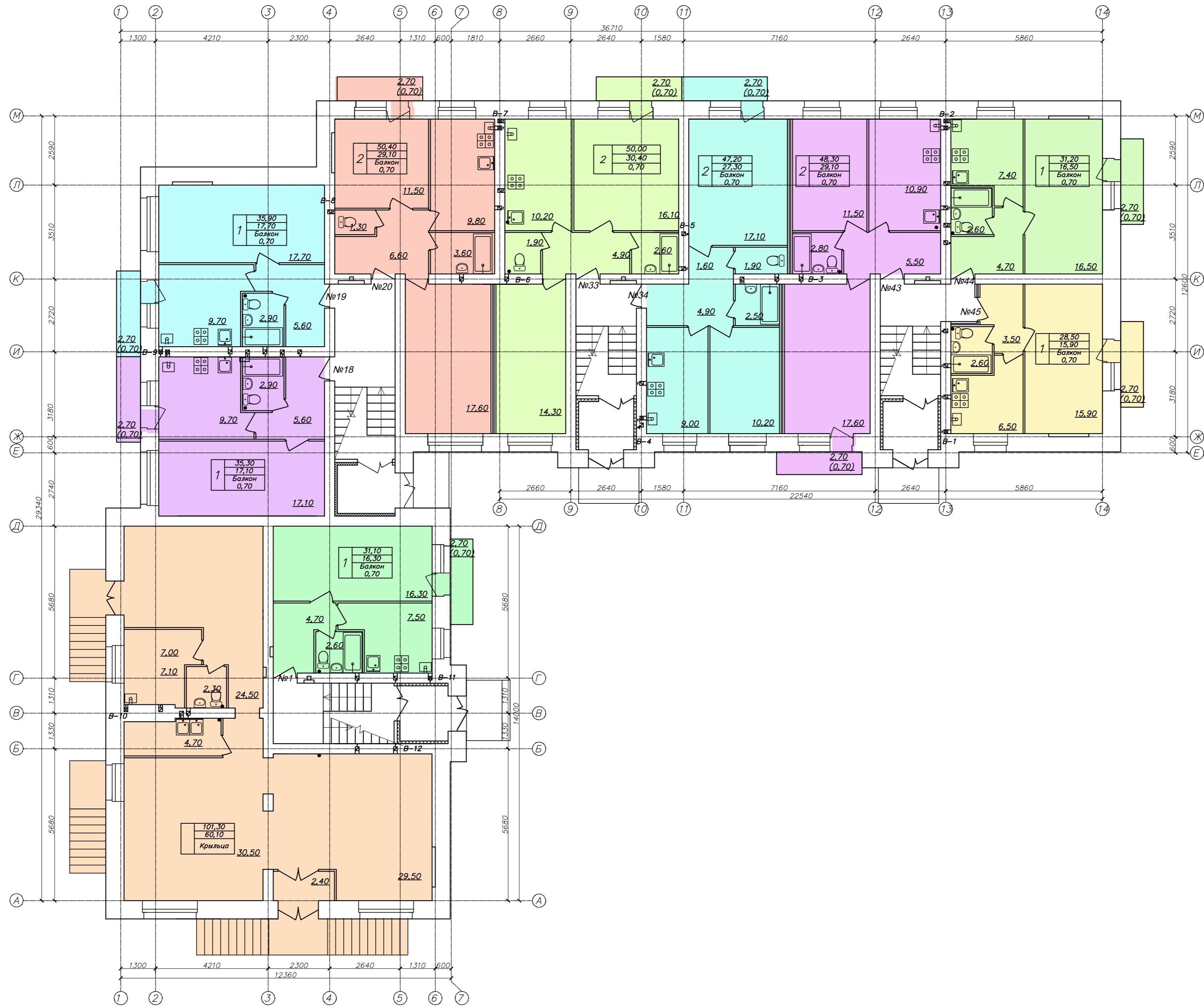
Кладочный план 1-го этажа.
